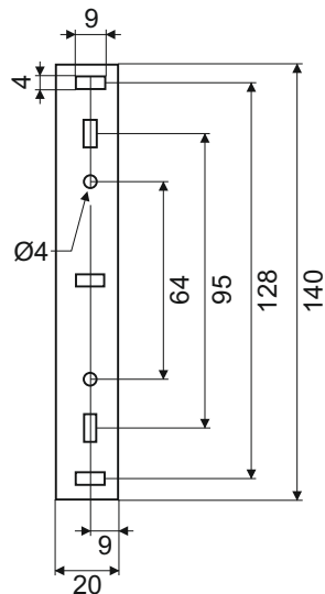
Монтажна планка / Door bracket
