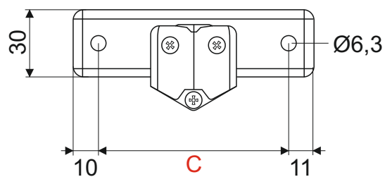
Монтажна планка Door bracket
