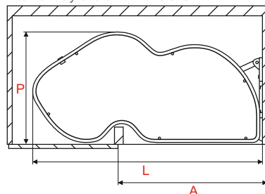
Размери при прибран бърбек Internal tray overall dimensions
