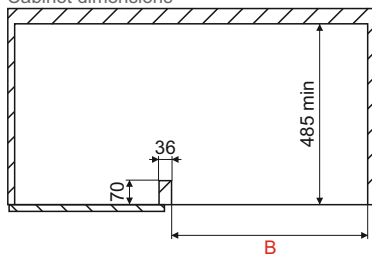
Размери на шкаф Cabinet dimensions
