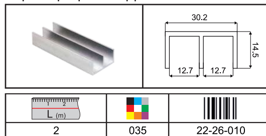
Горен профил - Upper rail
