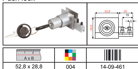
Ключалка Push lock
