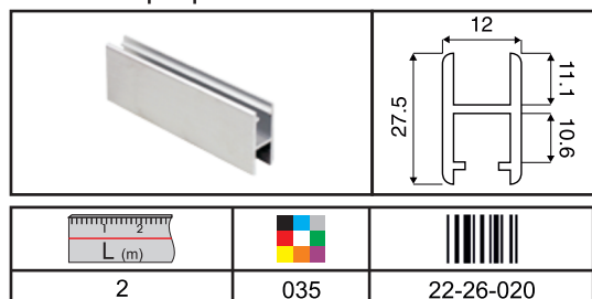
Релсов профил - Glass H-rail
