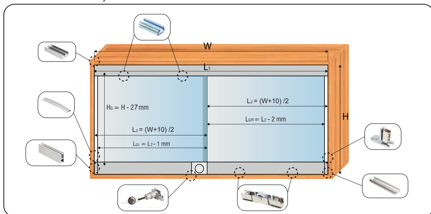
Схема на системата - System scheme
