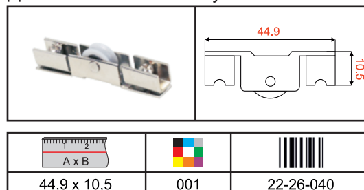
Долна количка - Trolley
