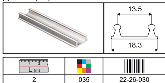
Долен профил - Down rail
