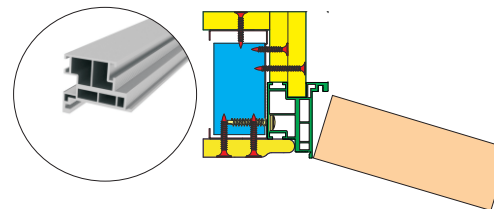
2 АЛУМИНИЕВ ПРОФИЛ VISIO 40 ВЪНШЕН
