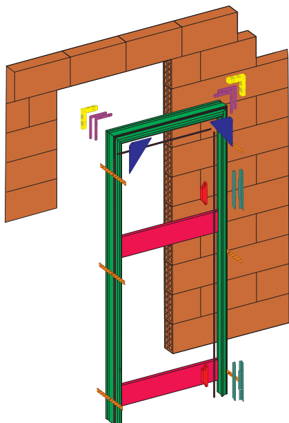
1 АЛУМИНИЕВ ПРОФИЛ VISIO 40 ВЪТРЕШЕН
